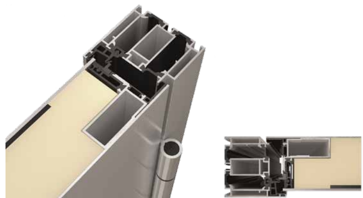
WB beidseitige Aufsatzfüllung Wohnbauflügel mit beidseitiger Aufsatzfüllung
