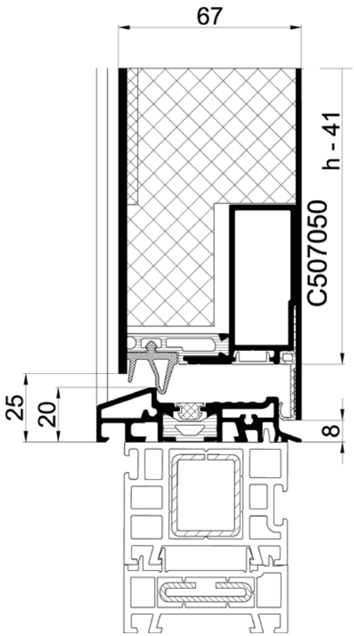
Schwellenansicht Wohnbauflügel
