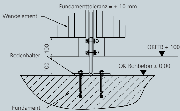
Detail 1 Bodenanschluss mit Fundamentdetail
