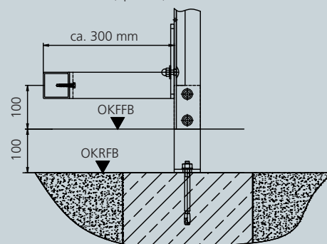
Schnitt 4-4 Rammschutz (optional)
