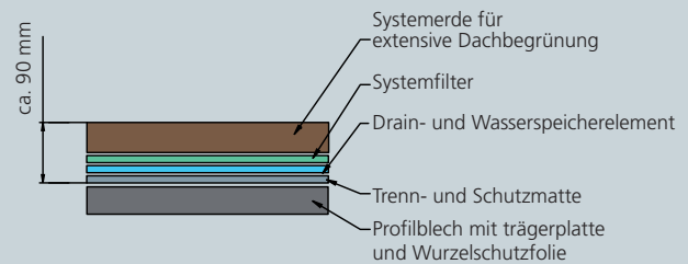
Schnitt Gründach (optional)
