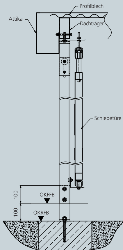
Schnitt 3-3 Schiebetüre und Attika
